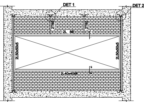
نمای وادارهای قائم و شیب درگامی ها در دیوارهای پیرامونی با بازشوی یکسره
