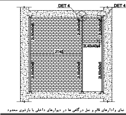
نمای وادارهای قائم و شیب درگامی ها در دیوارهای داخلی با بازشوی محدود
