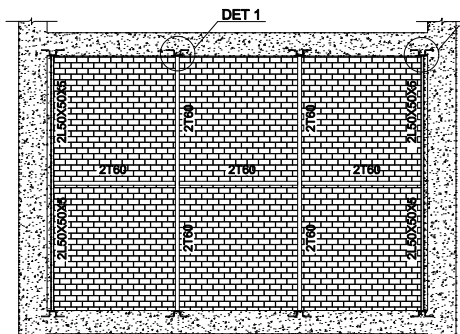
نمای وادارهای افقی و قائم دیوارهای پیرامونی در دهانه های بزرگتر از ۶ متر
