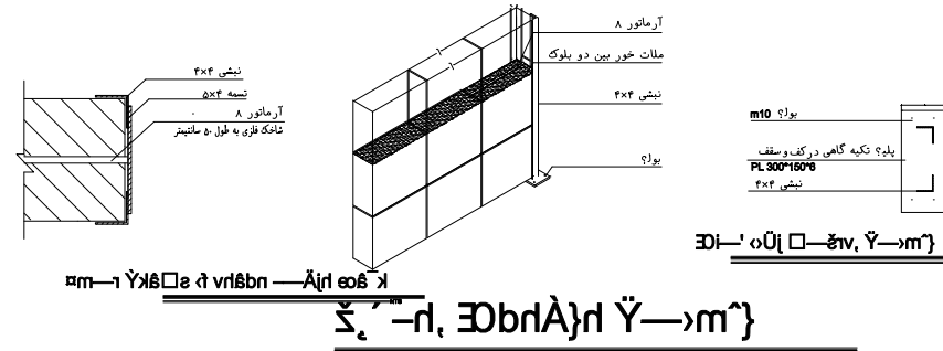
نمای وادارهای افقی و قائم دیوارهای داخلی در دهانه های بزرگتر از ۶ متر
