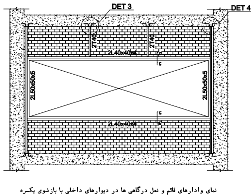
نمای وادارهای قائم و شیب درگامی ها در دیوارهای داخلی با بازشوی یکسره
