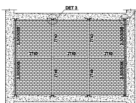
نمای وادارهای افقی و قائم دیوارهای داخلی در دهانه های بزرگتر از ۶ متر
