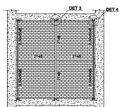
نمای وادارهای افقی و قائم دیوارهای داخلی در دهانه های کوچکتر از ۶ متر
