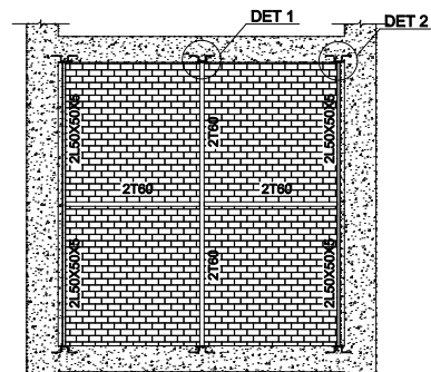
نمای وادارهای افقی و قائم دیوارهای پیرامونی در دهانه های کوچکتر از ۶ متر
