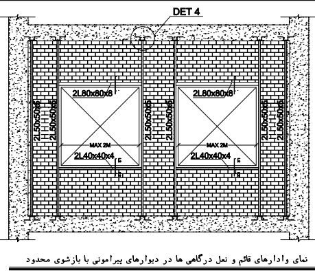
نمای وادارهای قائم و شیب درگامی ها در دیوارهای پیرامونی با بازشوی محدود
